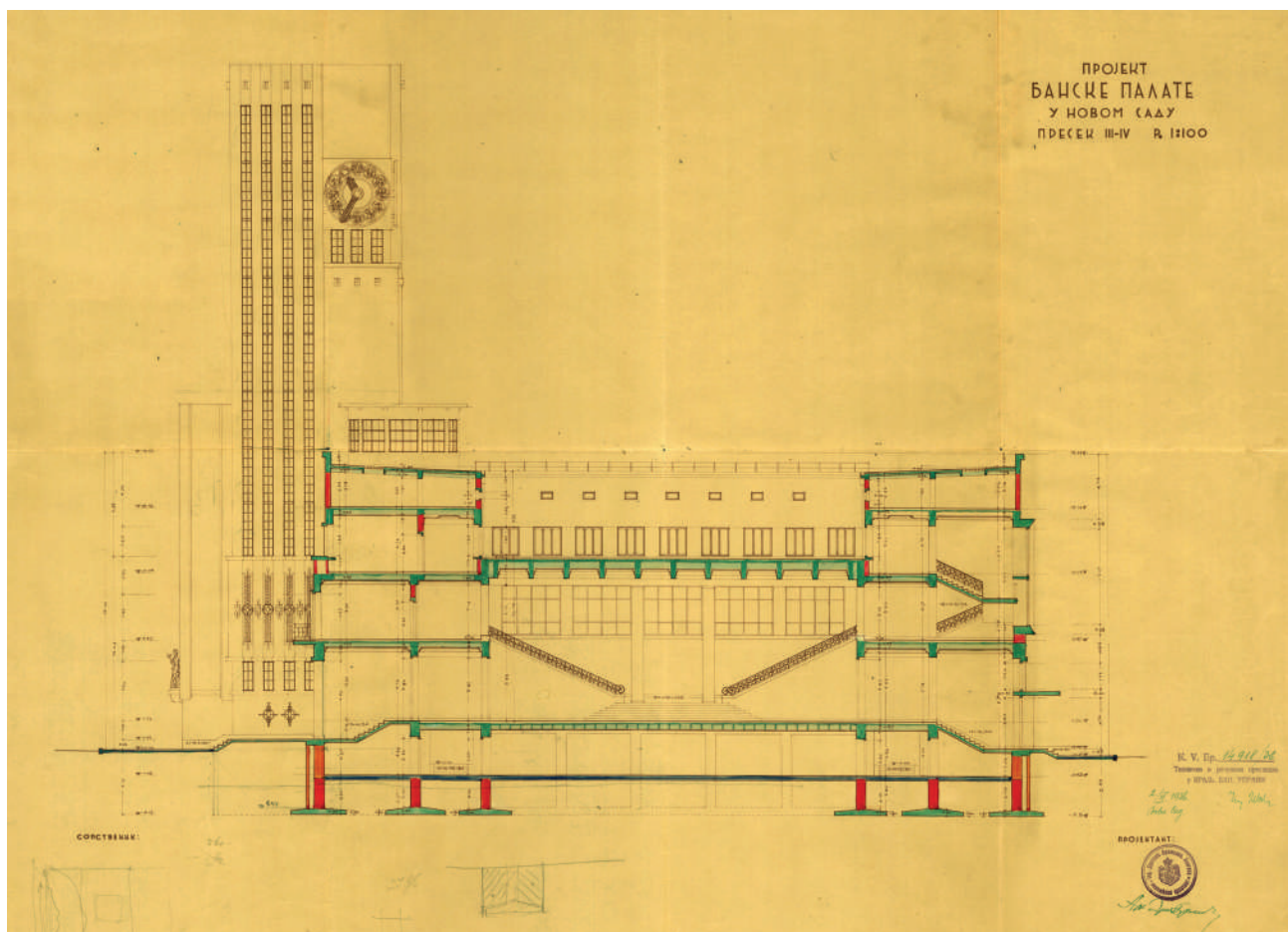
1936, јуни 2, Нови Сад. Део архитектонског пројекта Банске палате, Административна зграда, пресек кроз главни улаз III-IV , размера 1:100
