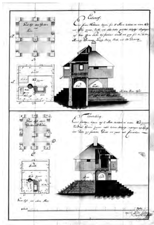
План граничарског чардака Извор: ИАБ-1184 – Збирка планова и мапа
