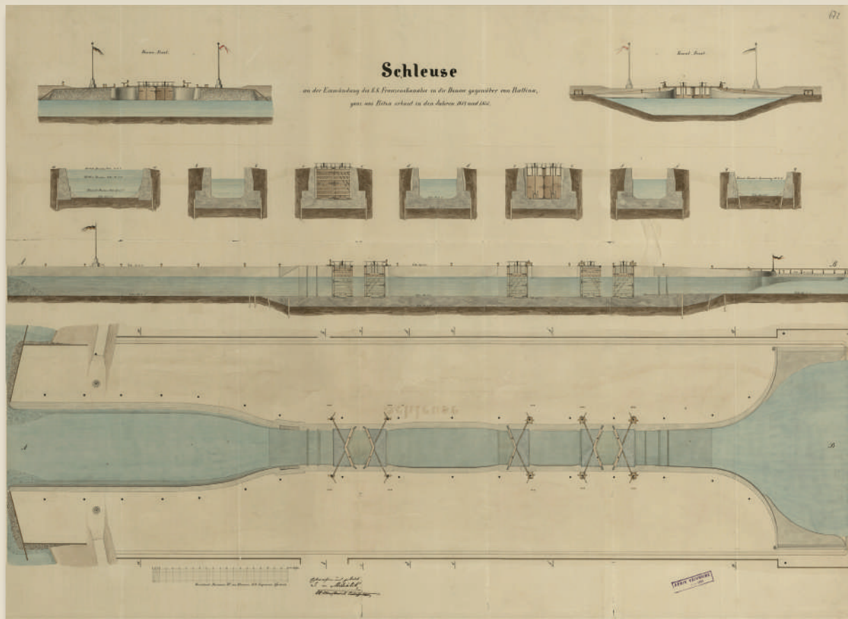
1856, Темишвар. Шлајз на уливу Францовог канала у Дунав насрам Батине, изграђен у потпуности од бетона 1854/55. године. (АВ, Ф. 23, През. сп., а. ј. 11727)
