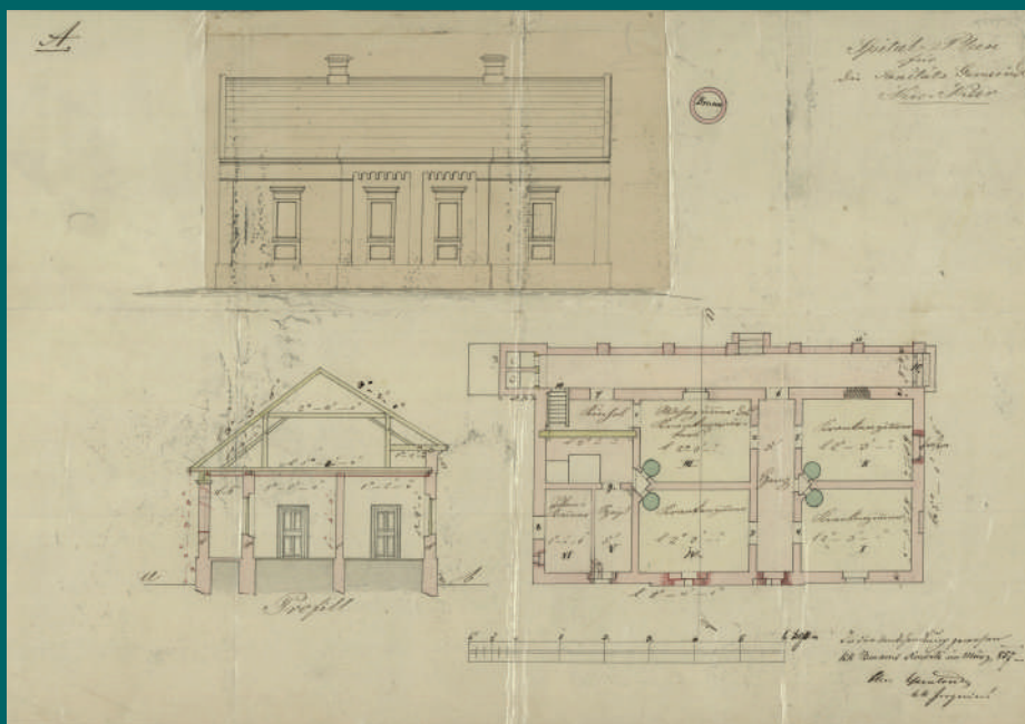
1857, Н. Сад. План болнице у Малом Керу (Бачко Добро Поље). (АВ, Ф. 373, а. ј. 360)
